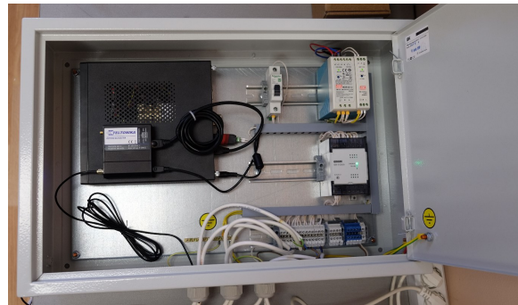
Шкаф опросной станции с безвентиляторным ПК со SCADA-сервером, промышленным роутером GSM/Ethernet/Wi-Fi, блоками питания и сетевым преобразователем USB-RS485(Modbus)
