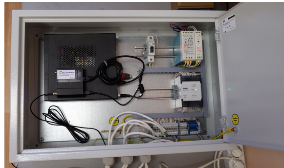
Шкаф опросной станции с безвентиляторным ПК со SCADA-сервером, промышленным роутером GSM/Ethernet/Wi-Fi, блоками питания, модулем ввода сигналов 8 каналов и сетевым преобразователем USB-RS485(Modbus)
