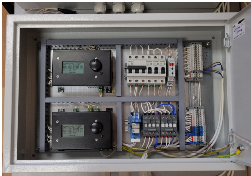
Шкаф горелочного устройства на 2 горелки с золоудалением и защитой по давлению и температуре теплоносителя
